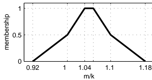
Figure 13: Fuzzy parameter m/k .
